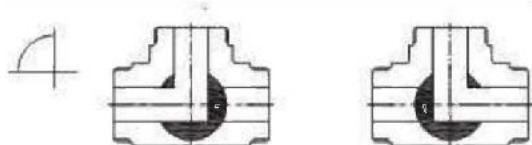
L型通口 L type gateway A向入口(A inlet) 90° 旋转方向(90 rotation direction)
